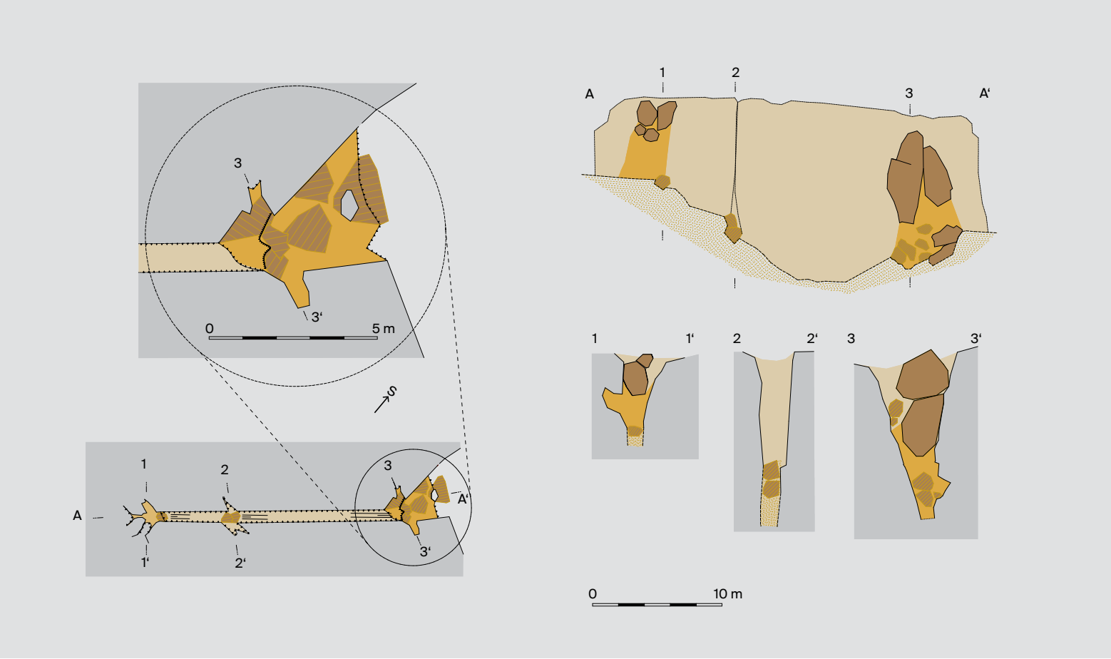
Jeskyně V Kuchyni (půdorys a základní řezy). Kreslil a mapoval: V. Ouhrabka, 2014
